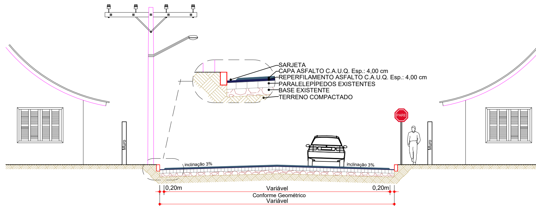
SEÇÃO TRANSVERSAL ESCALA:1/100
