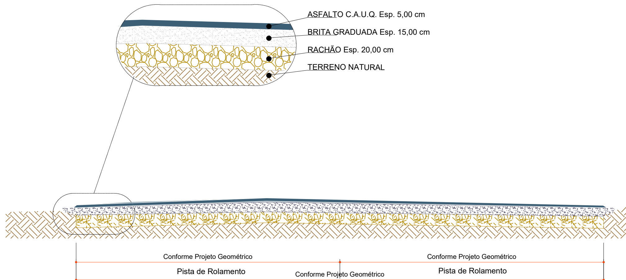
SEÇÃO TRANSVERSAL A SER EXECUTADA COM ASFALTO NOVO ESTACA 29+6.338 m ATÉ 36+1.698 m ESCALA: 1/40
