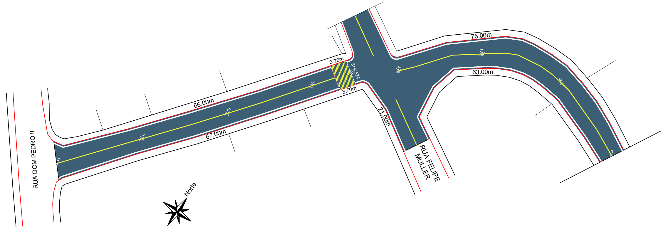
PLANTA SINALIZAÇÃO ESTACA 0.P.P ATÉ 7 ESCALA: 1/500
