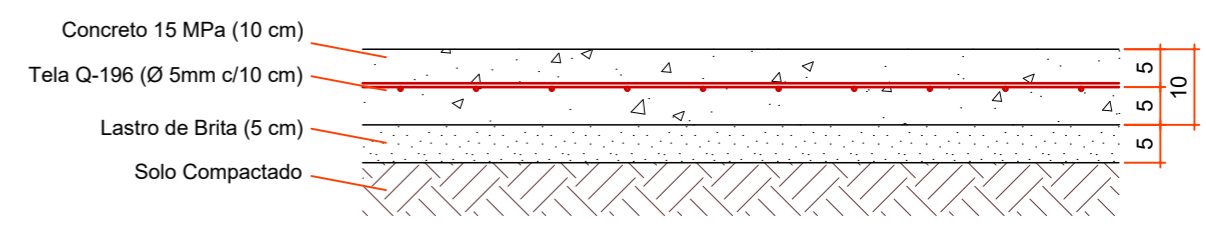
DETALHE DO PISO ESC 1:10
