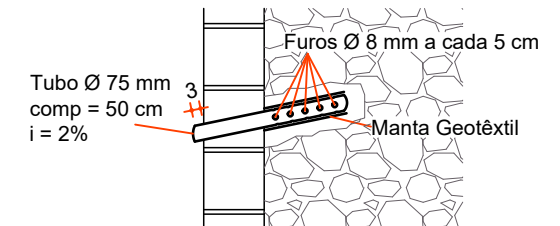
DETALHE BARBACÃ ESC 1:25
