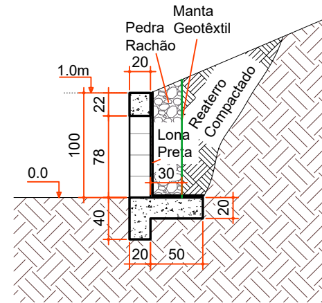
CORTE B-B ESC 1:50
