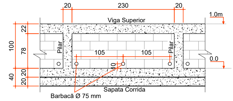
VISTA FRONTAL ESC 1:50
