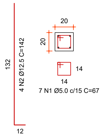
PILARES ESC 1:25
