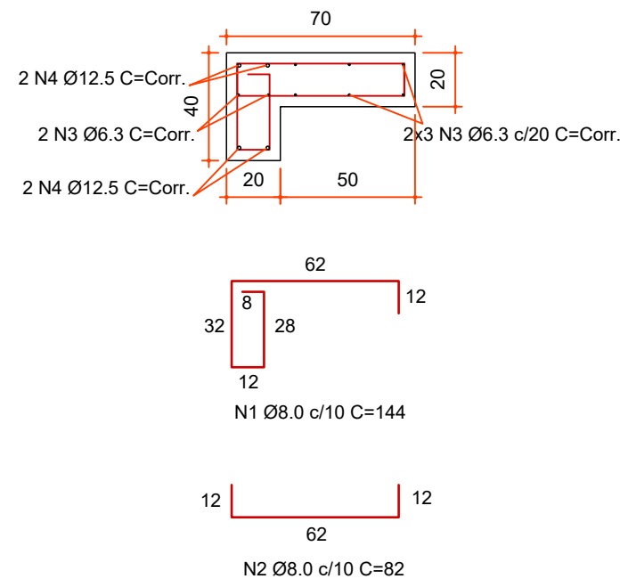
SAPATA CORRIDA ESC 1:25
