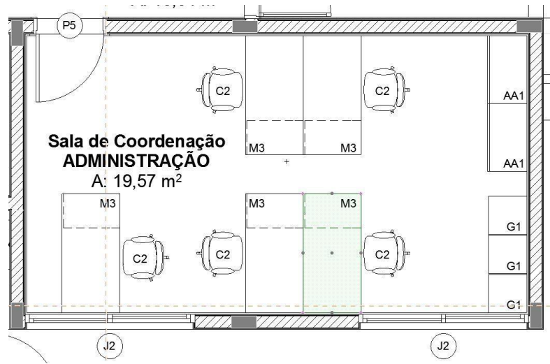
Figura 12 – Planta baixa da Sala de Coordenação
