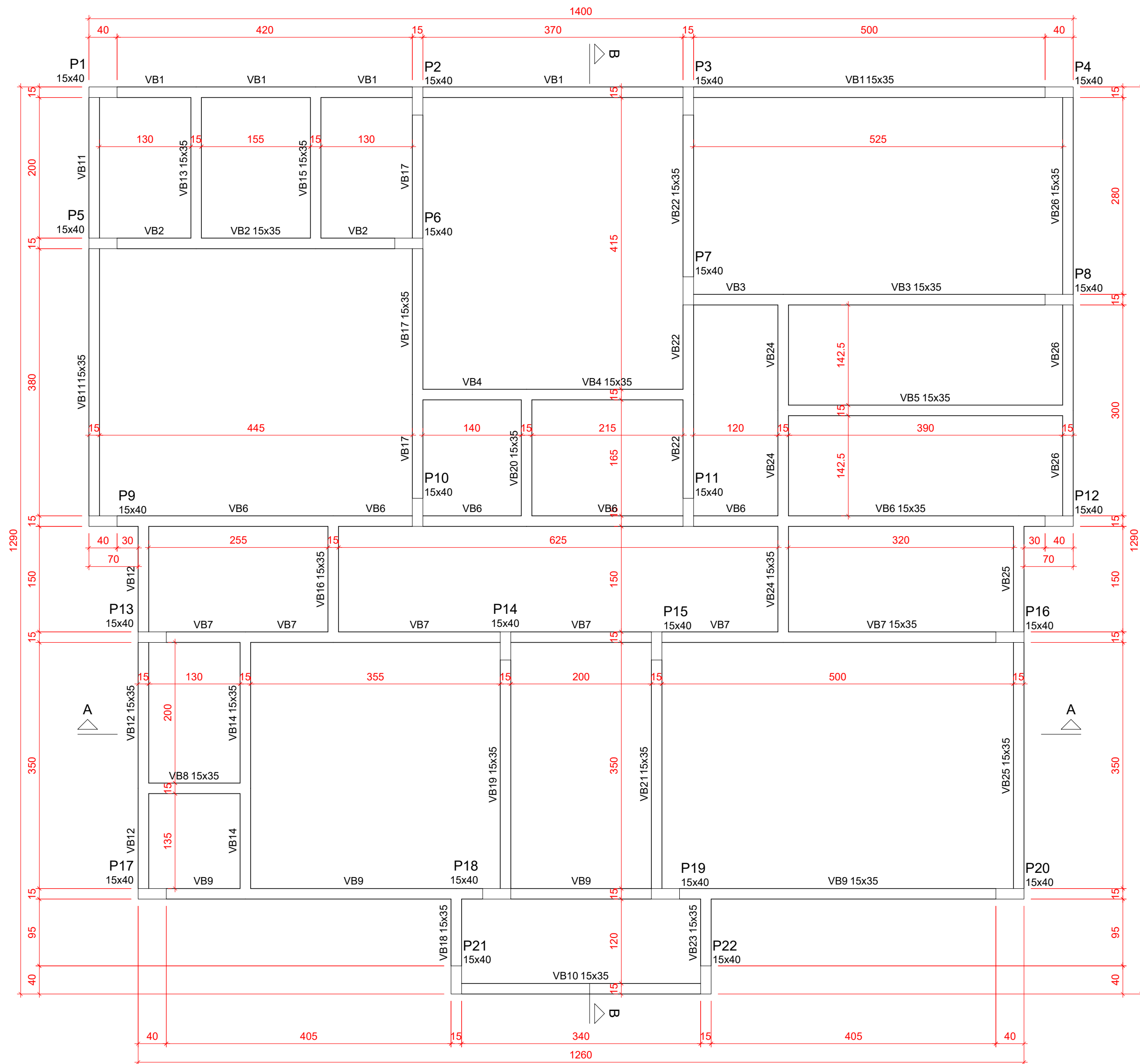
Planta de Formas do Baldrame (Nível 0) escala 1:50
