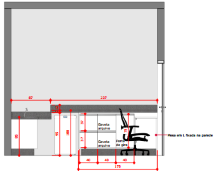
VISTA 03 ESCALA: 1/10
