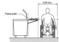
Figura 136 - Refeitórios - Medidas e espaço para circulação - Vista frontal
