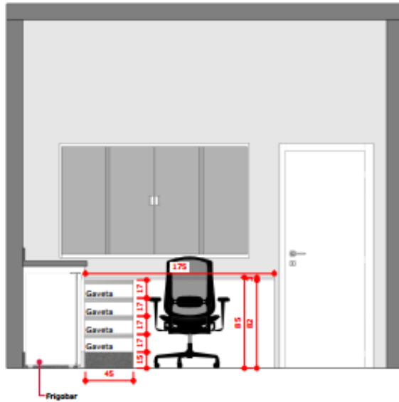
VISTA 02 ESCALA: 1/10
