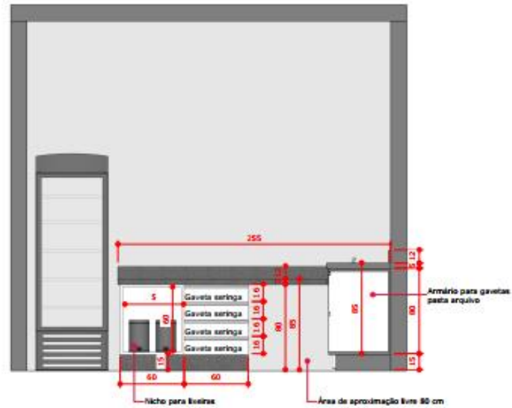
VISTA 01 ESCALA: 1/10
